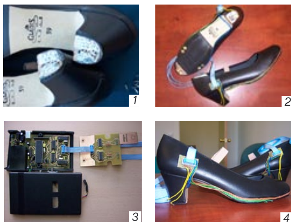
Fig. 1: Muestra de clavos de los tacones Fig. 2: Detectores de contactos Fig. 3: Dispositivo principal Fig. 4: Transceptor de comunicaciones
